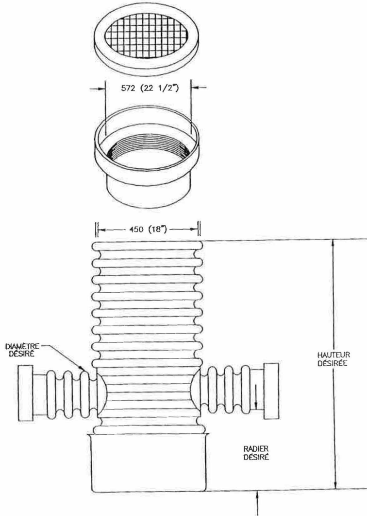
COUPE D-D PUISARD TYPE
